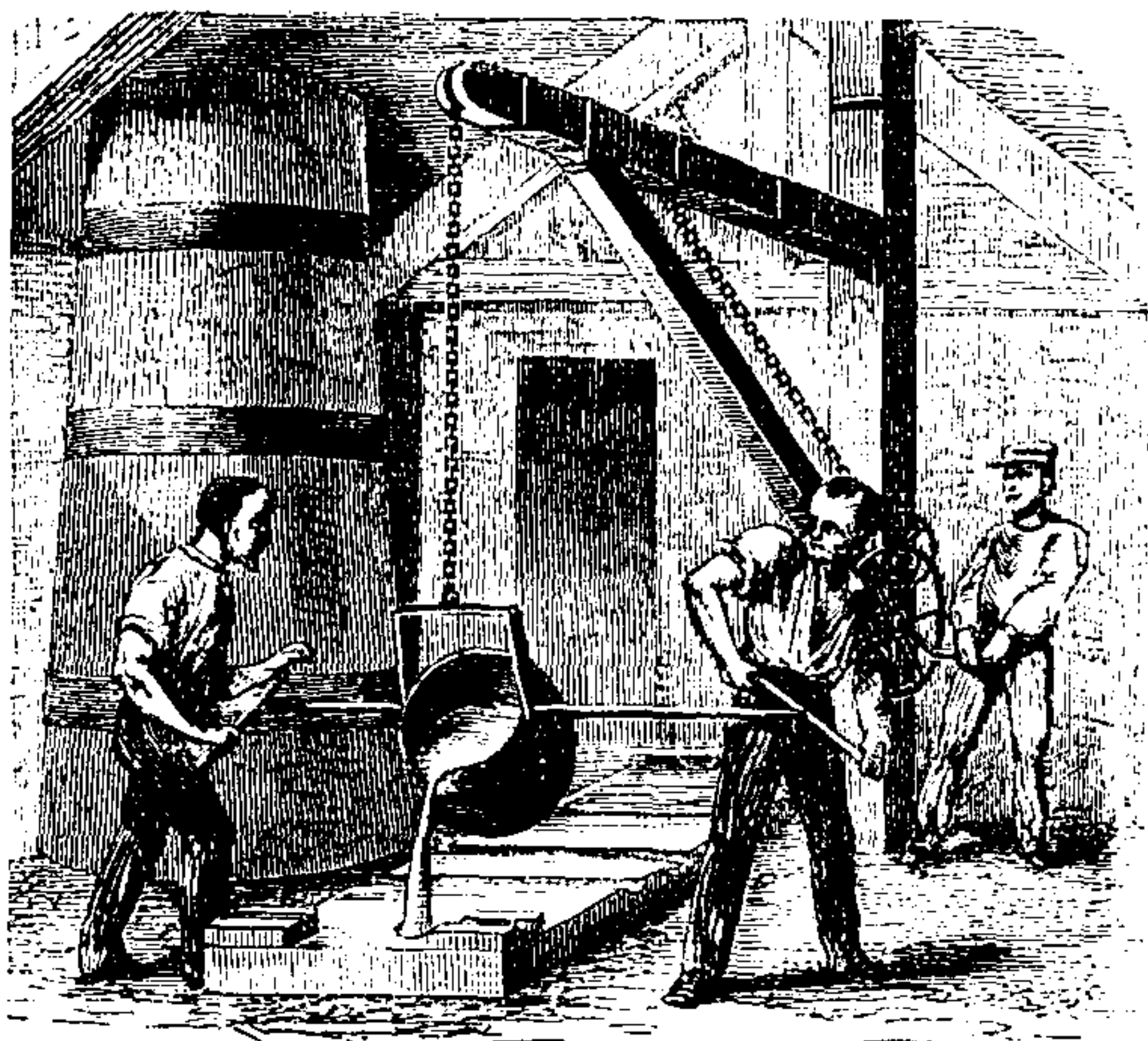
OUVRIERS COULANT LA FONTE DANS UN MOULE. — Cet énorme vase en tôle qui est suspendu à une grue et que manient à grand'peine deux ouvriers peut contenir des milliers de kilogrammes de métal fondu. On verse le métal dans une ouverture qui communique avec un moule creux placé sous la terre. Ainsi se fondent les cloches, les canons et tous les gros objets en fer ou en fonte.
