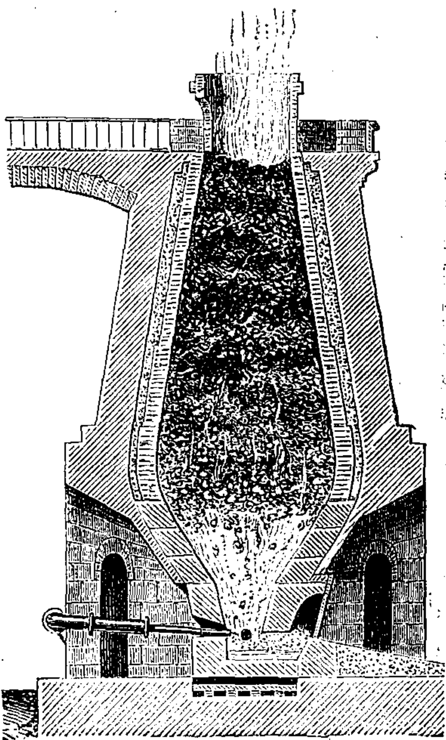
UN HAUT-FOURNEAU. — Les hauts-fourneaux sont des espèces de tours solides qu'on remplit par en haut de minéral de fer. Une fois que le haut-fourneau est allumé, on le remplit jour et nuit sans interruption pour avoir la plus grande chaleur possible, jusqu'à ce que les murs usés se fendent et éclatent. A mesure que le fer se fond, il tombe en dessous, dans un réservoir.
