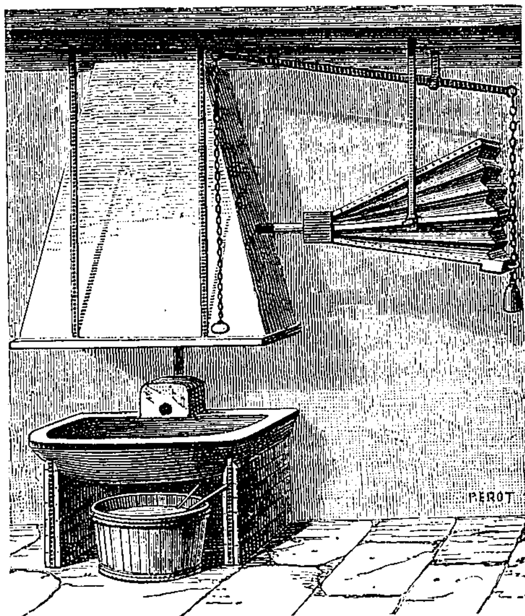
FORGE DE SERRURIER. — On voit derrière l'âtre un petit trou noir : c'est par ce trou qu'arrive le vent du soufflet, qui sert à exciter le feu de charbon de terre. Au-dessous du foyer se trouve un baquet rempli d'eau ; on s'en sert pour mouiller le charbon.
