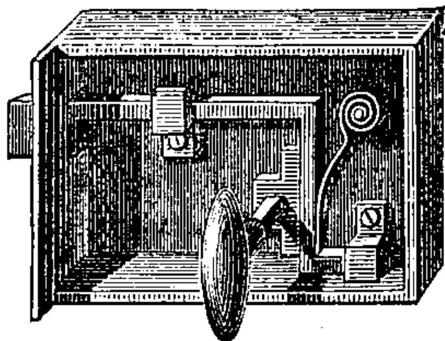
SERRURE APPELEE BEC DE CANE. — C'est la serrure la plus simple. Il suffit pour la fermer de pousser la porte ; le ressort qu'on voit à droite la maintient fermée.
