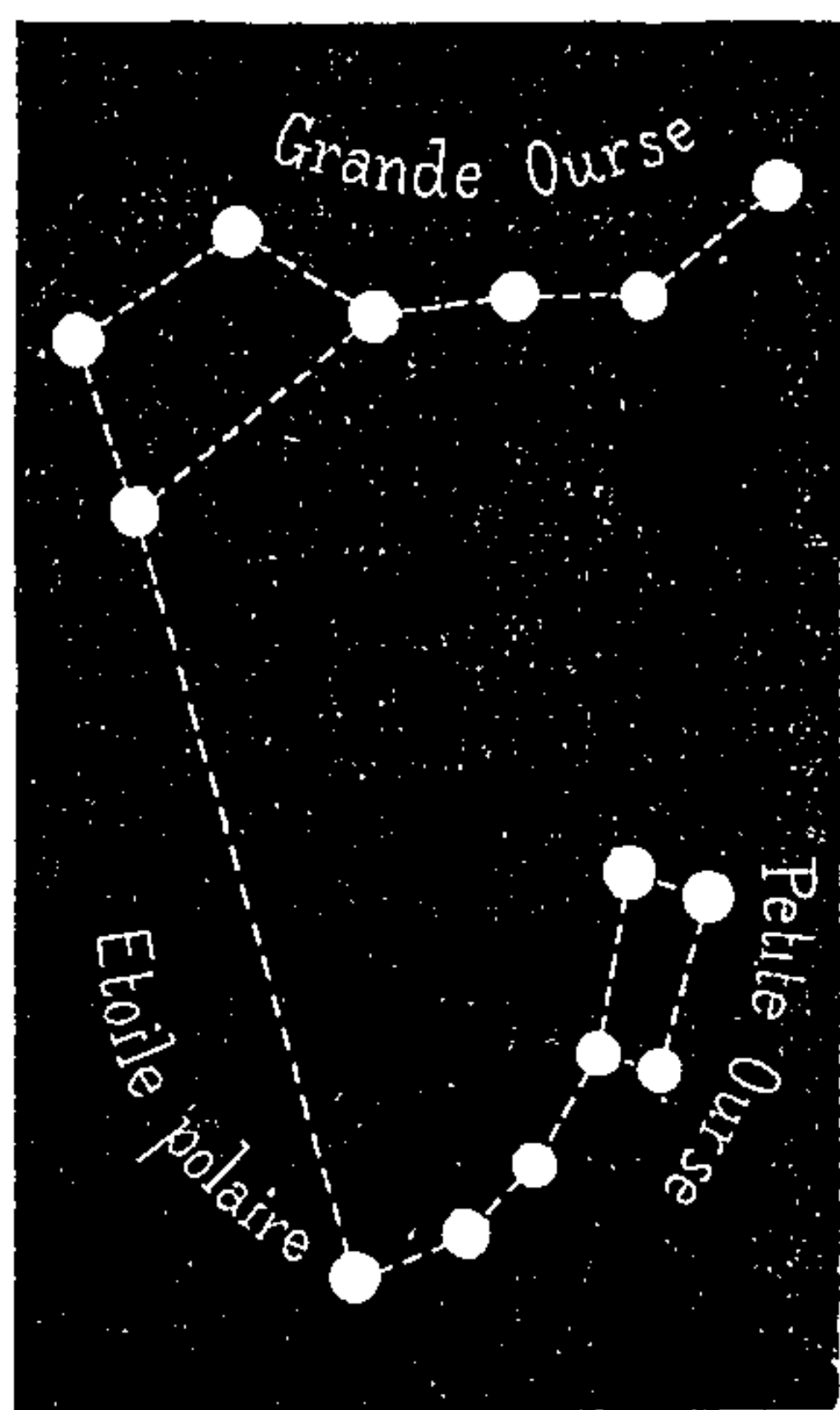
L'ÉTOILE POLAIRE ET LA GRANDE OURSE. — Il est utile d'apprendre à connaître dans le ciel les étoiles qui forment la constellation du grand Chariot ou grande Ourse . Près d'elles on aperçoit l'étoile polaire qui marque exactement le nord et indique la nuit les points cardinaux.
